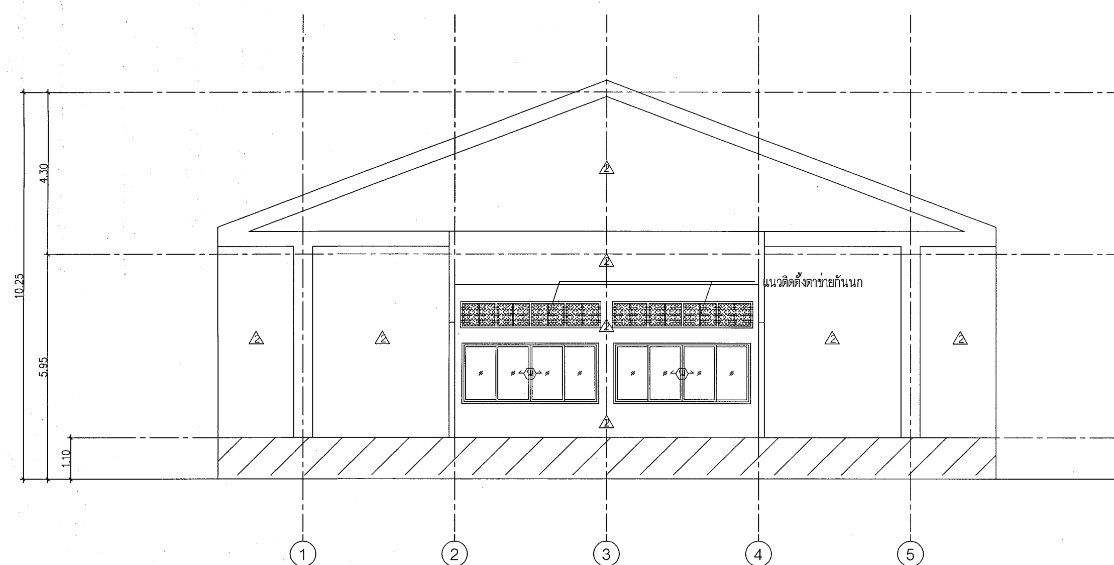
รูปด้าน ② 1:100
