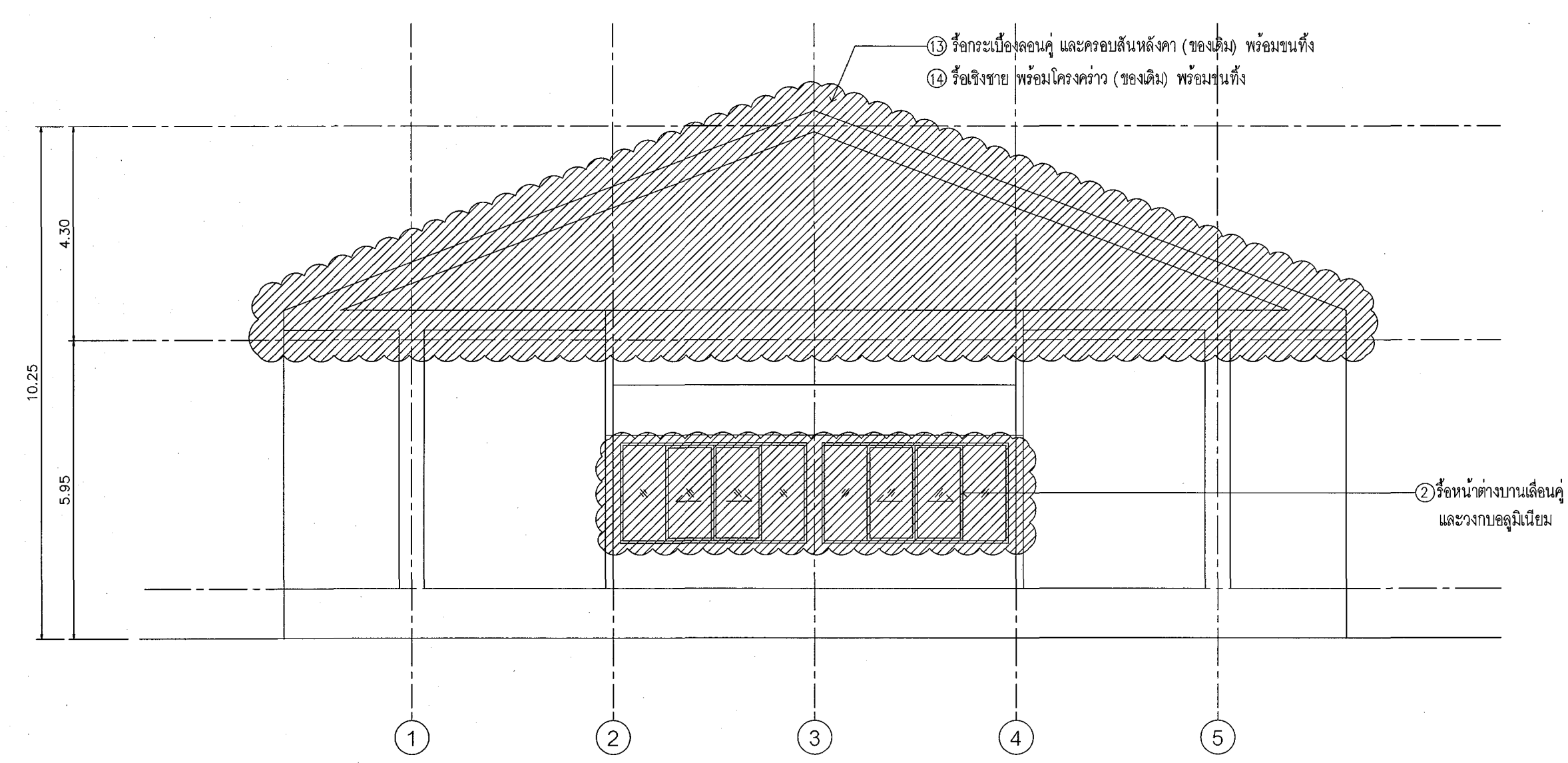
รูปด้าน ② มาตราส่วน 1:100
