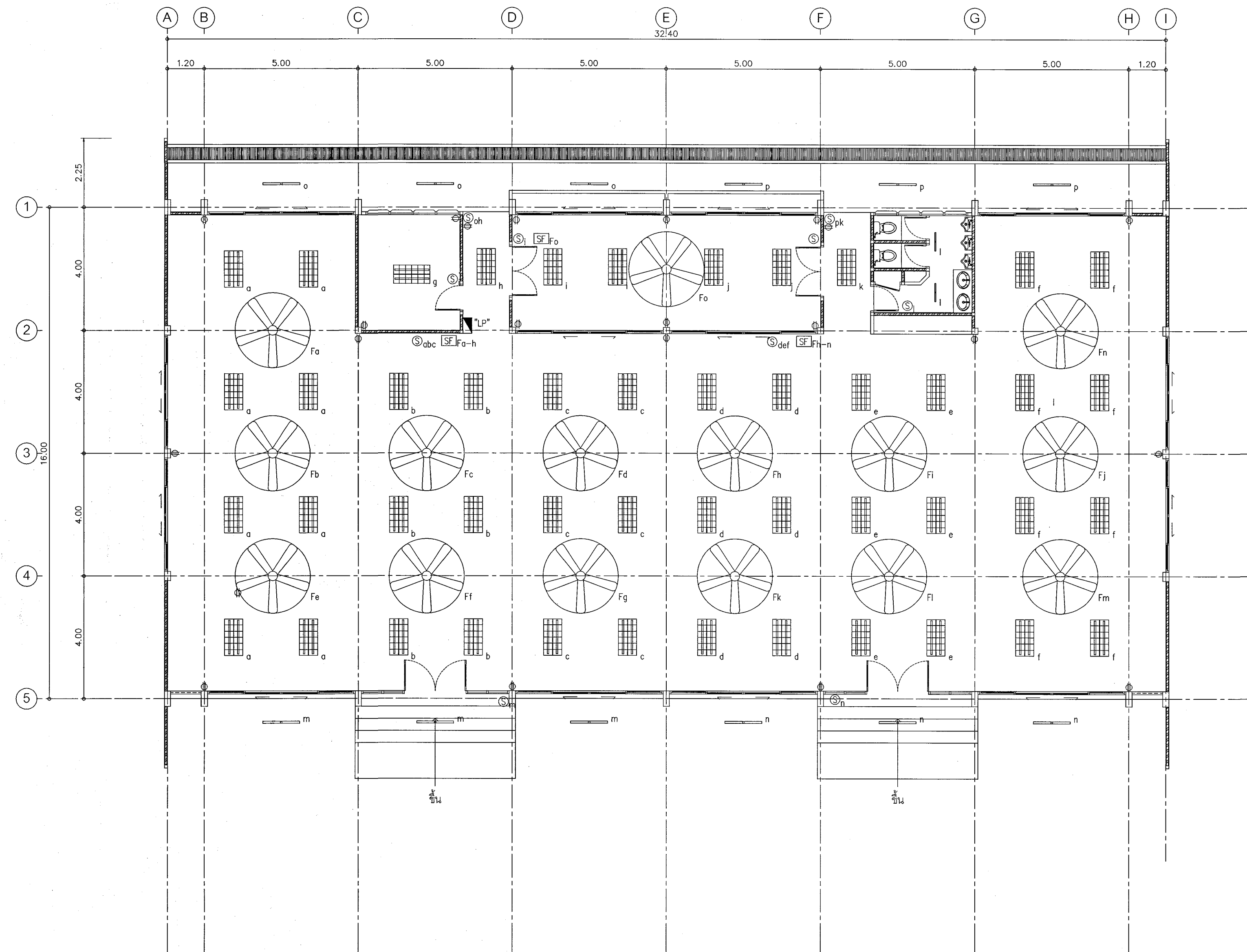
แปลนไฟฟ้า มาตราส่วน 1:100
