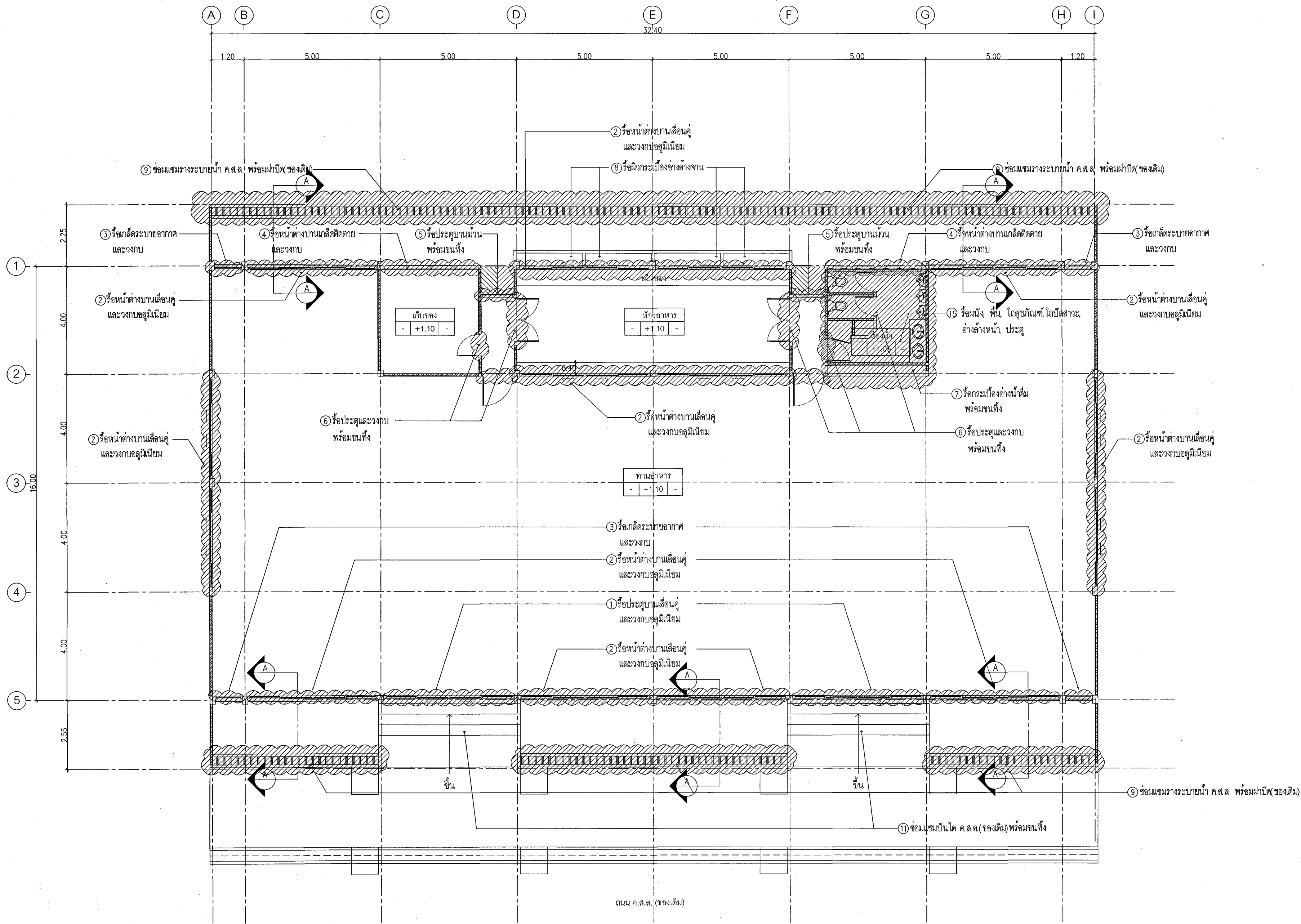
แปลน (รื้อถอนวัสดุ) มาตราส่วน 1:100
