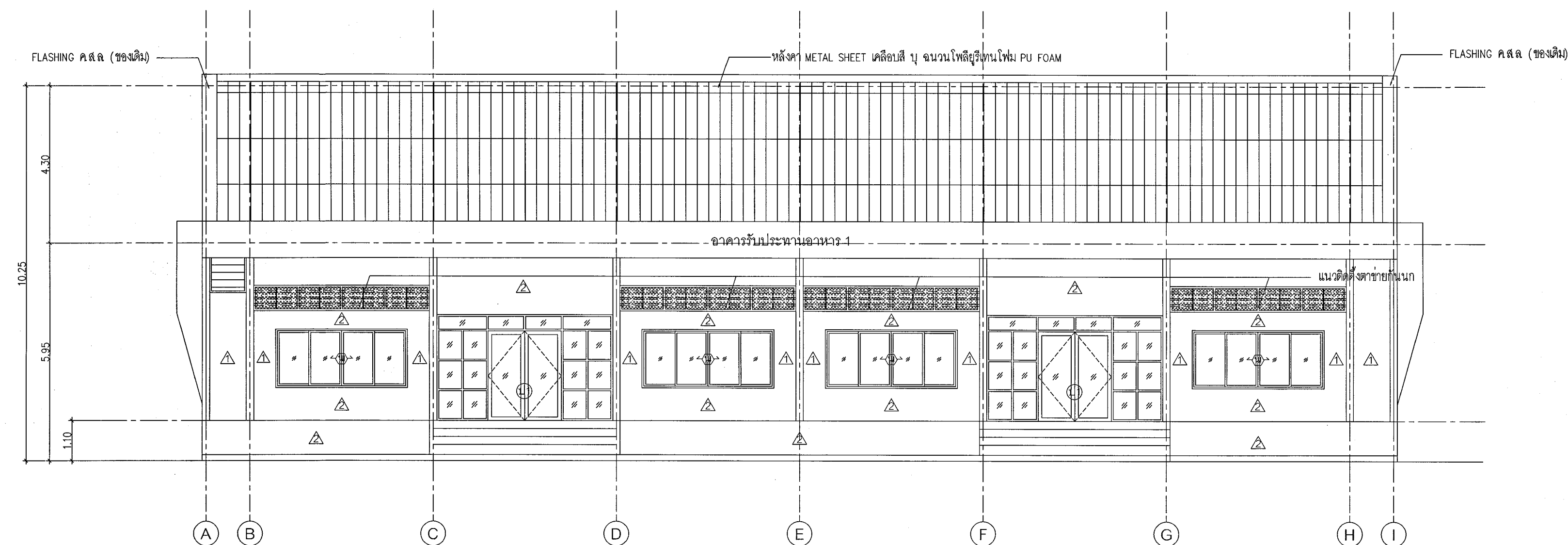
รูปด้าน ① 1:100
