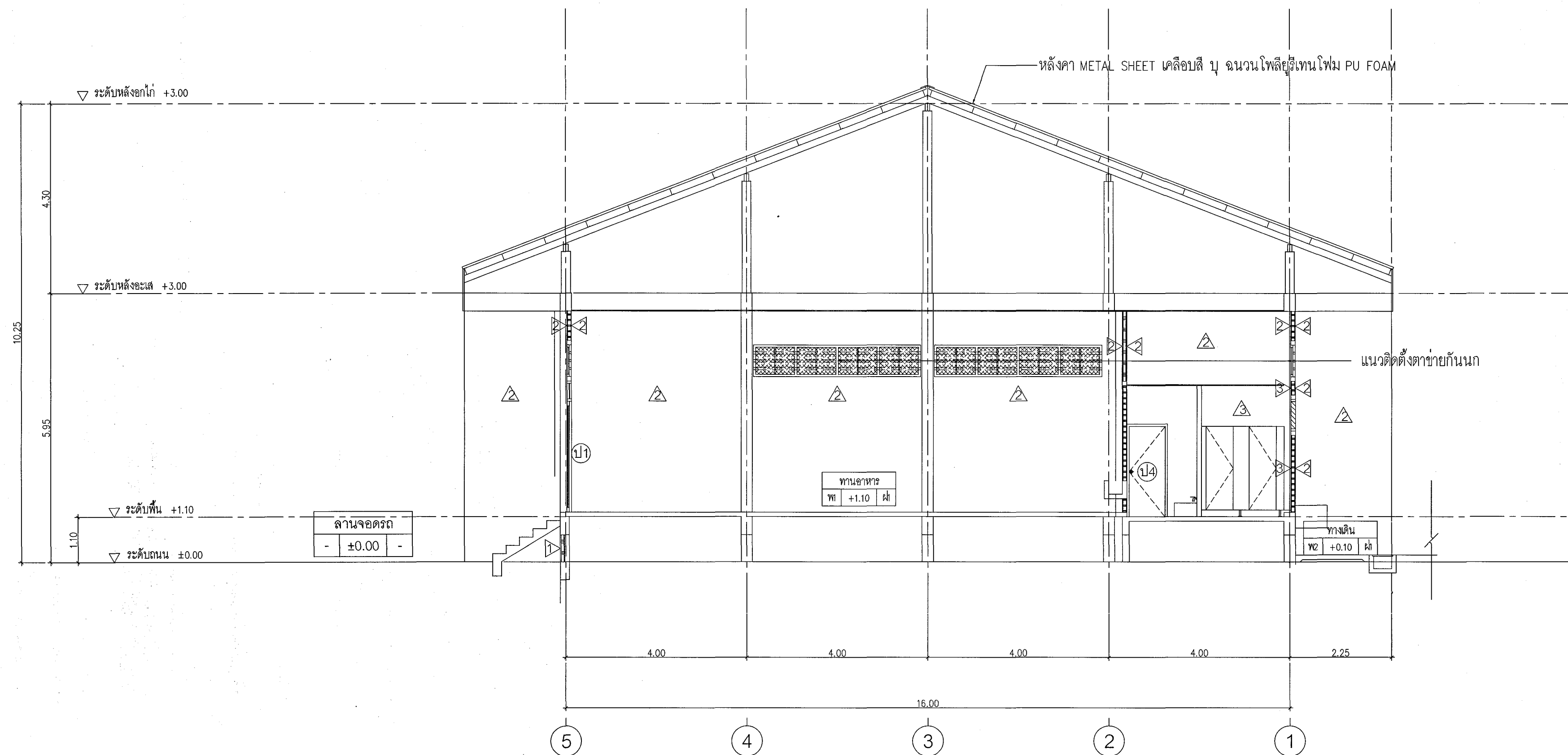
รูปตัด A 1:75
