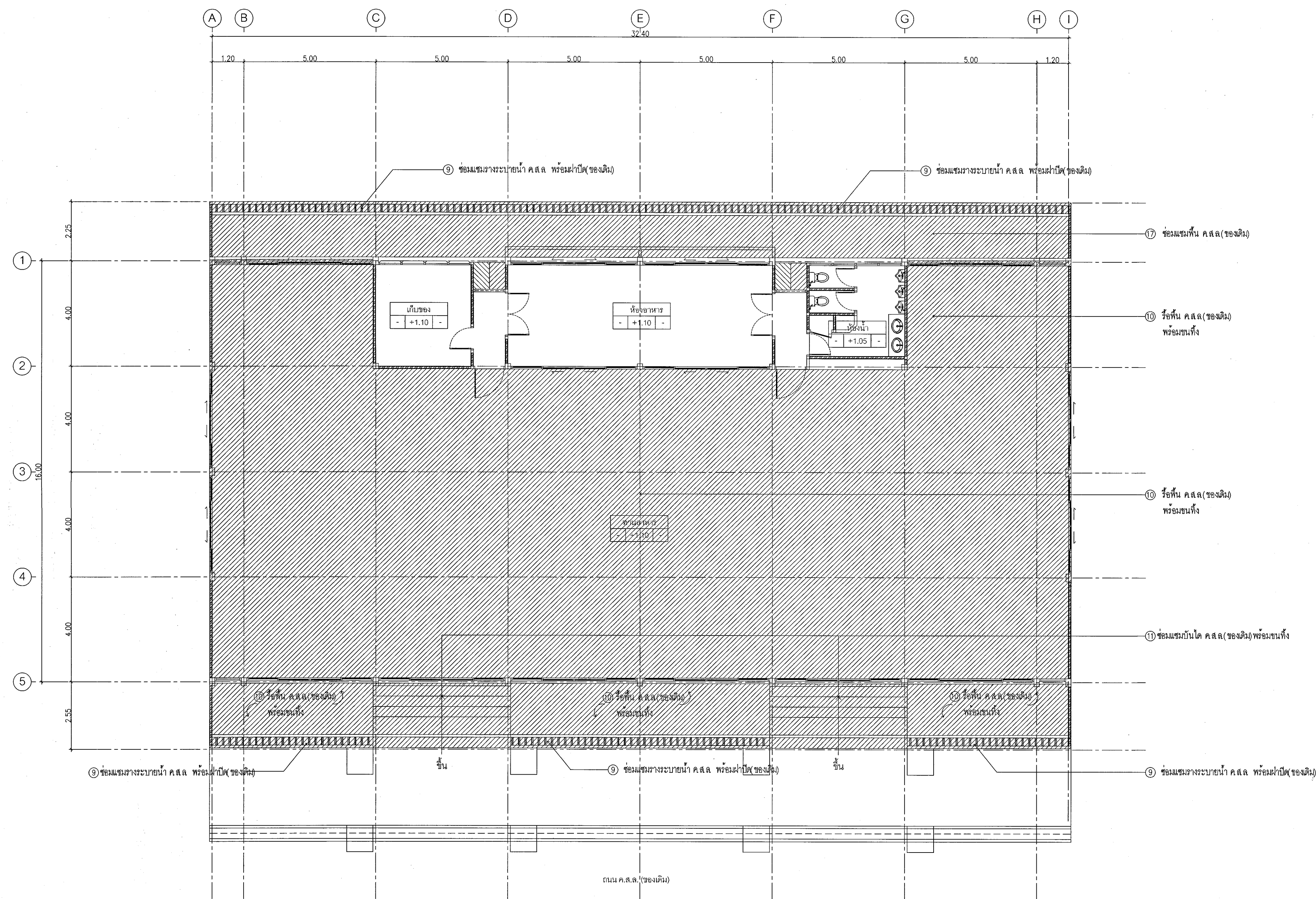
แปลนรื้อถอน พื้น ค.ส.ล. มาตราส่วน 1:100
