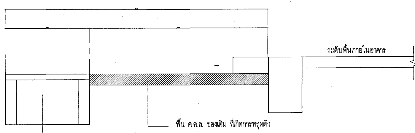
SECTION A-A ก่อนซ่อมแซม 1:20
