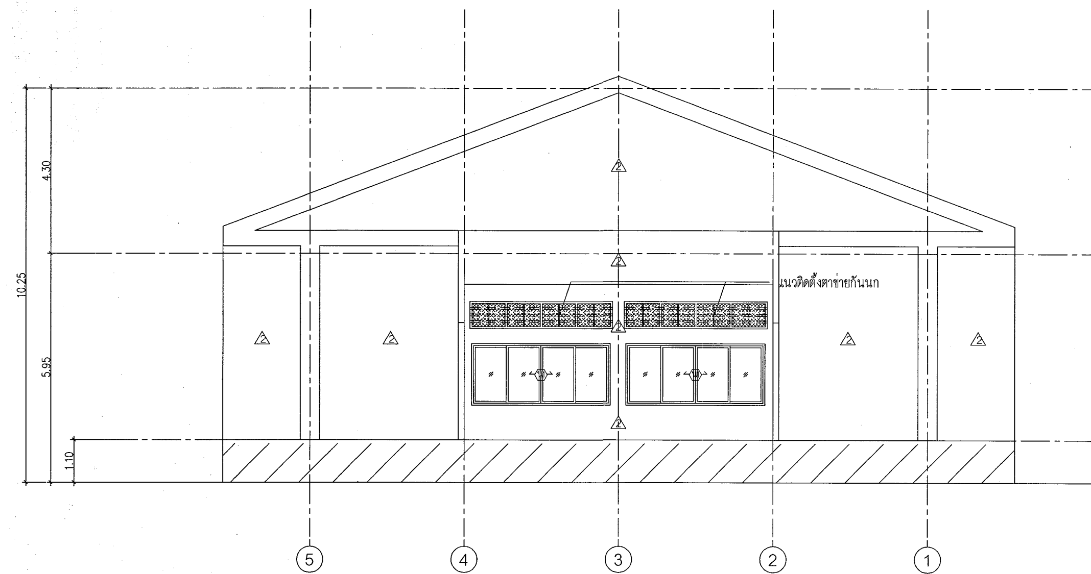
รูปด้าน ③ 1:100
