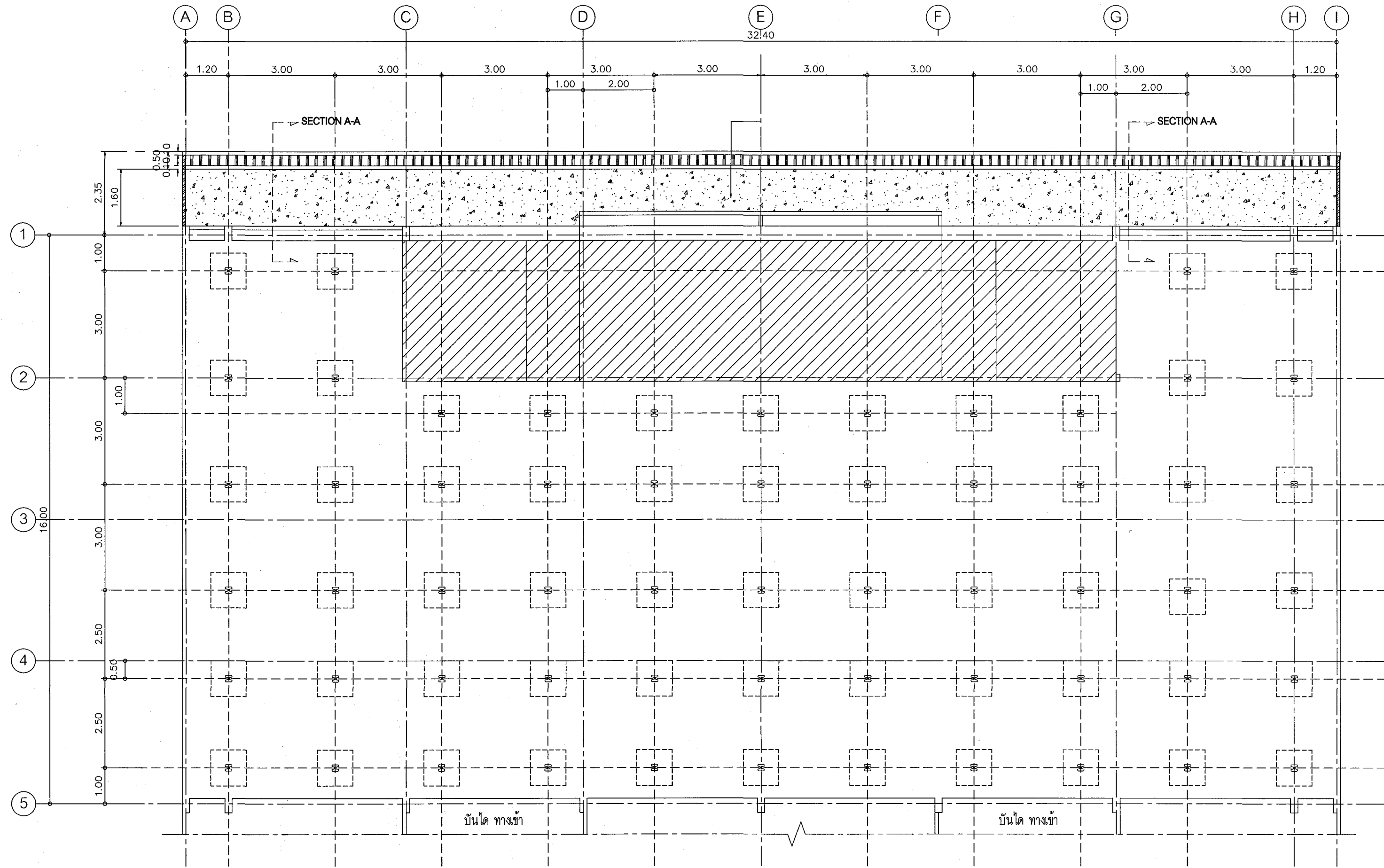
MICRO PILE I SECTION 0.18x0.18 m. จำนวน 59 ต้น
