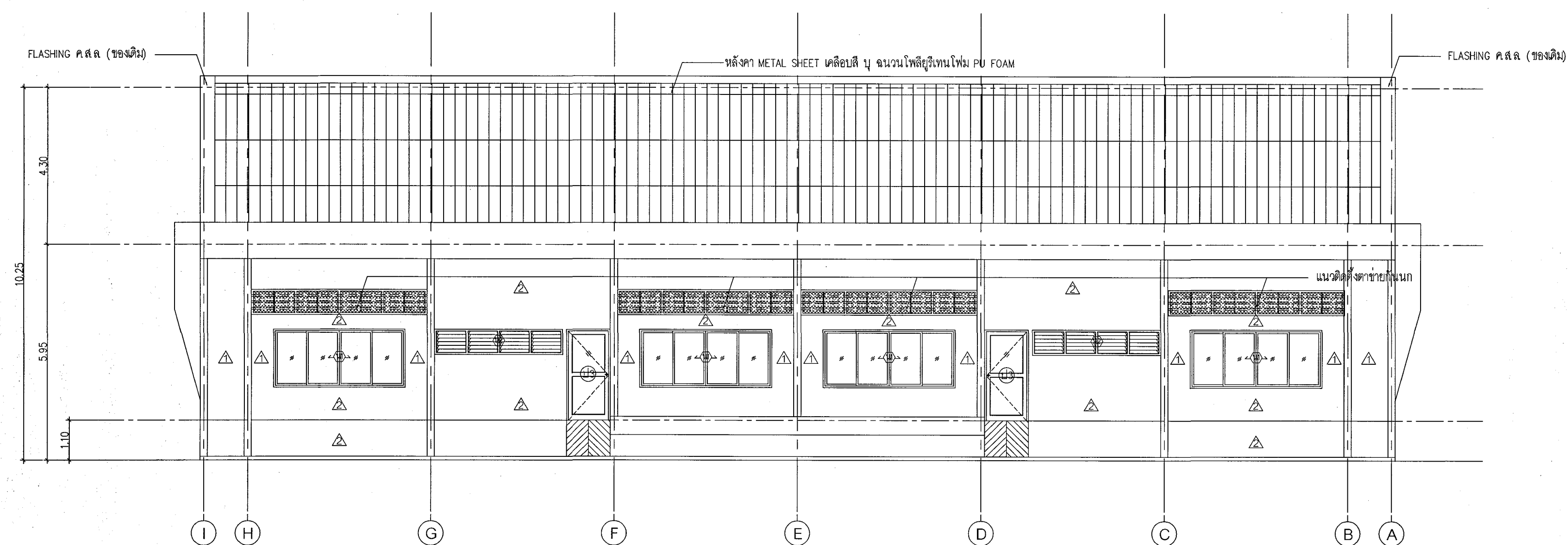
รูปด้าน ④ 1:100
